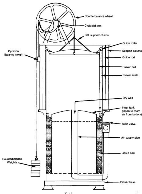
b. Bell Prover
